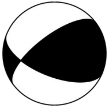
発震機構・モーメントテンソル図 https://www.fnet.bosai.go.jp/
