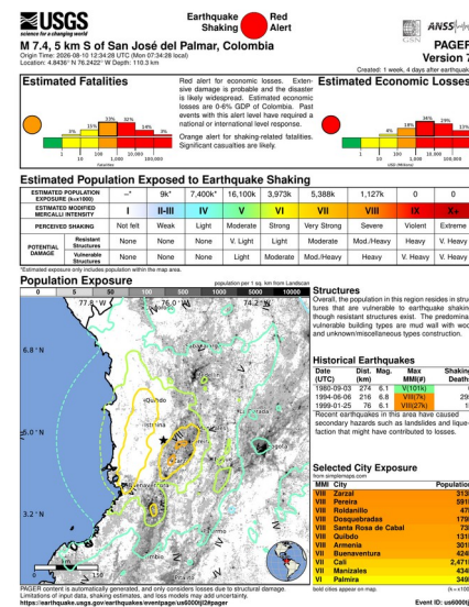
USGS PAGER 一枚図 (第 7 版) — 警報レベル・曝露人口・主要都市の曝露 https://earthquake.usgs.gov/earthquakes/eventpage/us6000tjl2/pager
