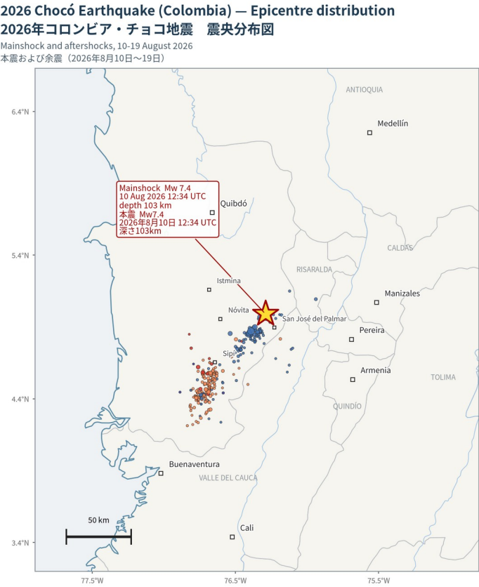
震央分布図: 本震および余震 284 回 (2026 年 8 月 10 ～ 19 日)。SGC 地震カタログ、地形は Natural Earth https://bdrsnc.sgc.gov.co/paginas1/catalogo/index.php
