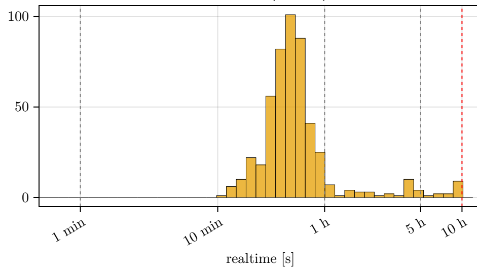
TRBDF2 (n=500)
