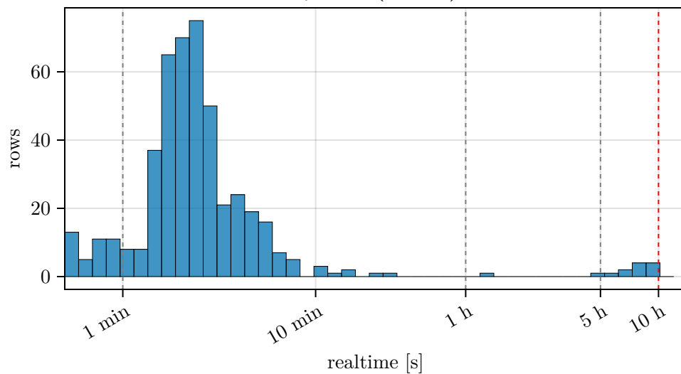
QNDF (n=500)
