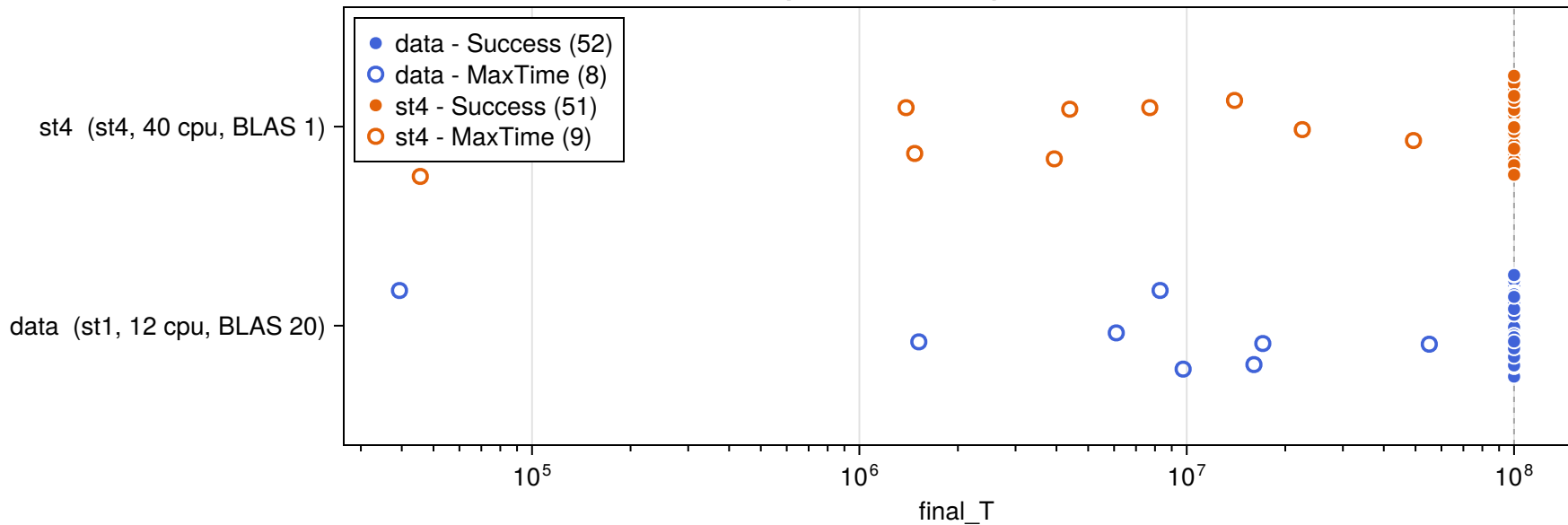
final_T per row, 60 rows per run (T = 1e+08)
