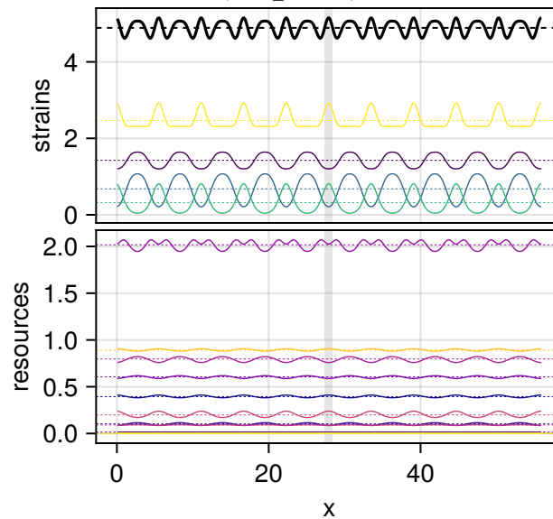
relamp 0.11, FWHM 0.02 L Success, final_T 1e+08 , maxresid 2.2e-13
