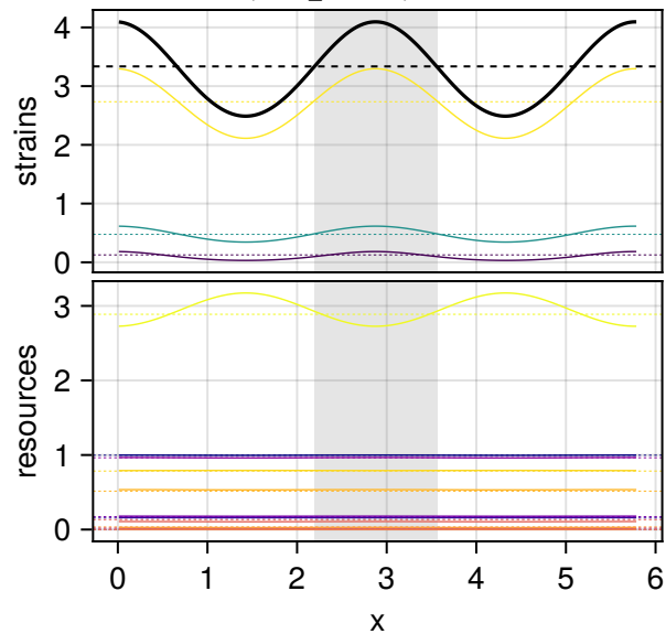
relamp 0.49, FWHM 0.24 L Success, final_T 1e+08 , maxresid 4.0e-12
