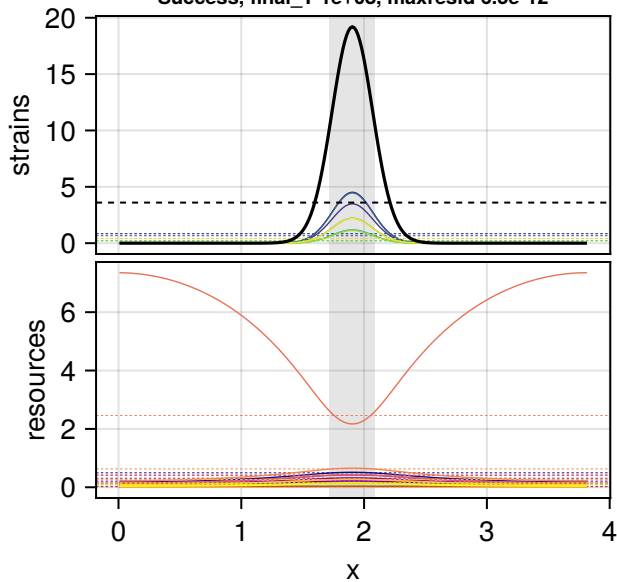
relamp 9.10, FWHM 0.10 L Success, final_T 1e+08, maxresid 6.5e-12
