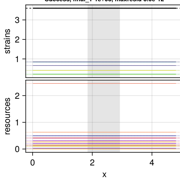
relamp 0.00, FWHM 0.23 L Success, final_T 1e+08, maxresid 3.0e-12
