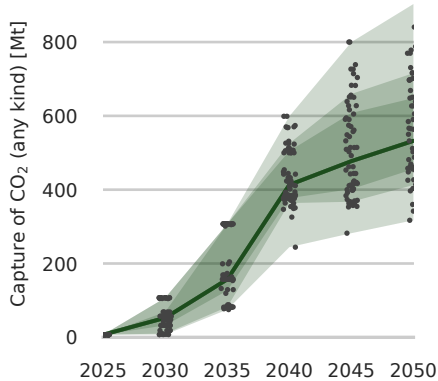
Cost-optimisations
