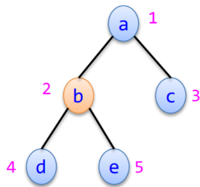
n=5 \Rightarrow n_1=0 ，最后 分支结点为 n/2=2
