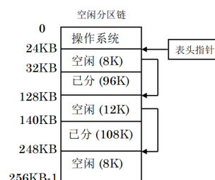
图 10: 空闲分区链
