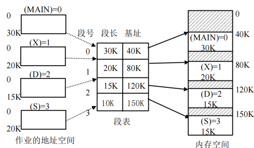
图 10: 分段管理示意图
