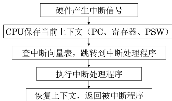
图 24: 中断处理程序示意图
