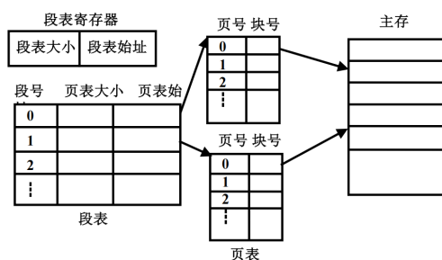
图 11: 段页式管理示意图
