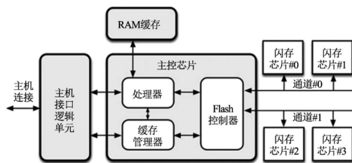
图 19: 固态硬盘结构示意图
