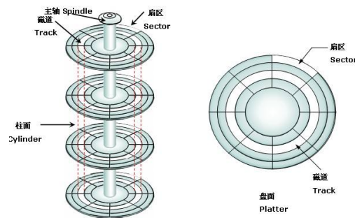
图 18: 机械硬盘结构示意图
