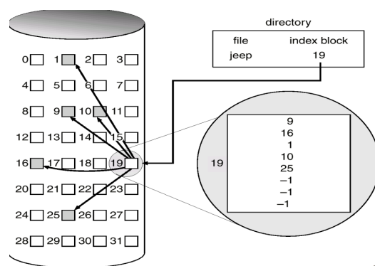
图 20: 索引分配示意图
