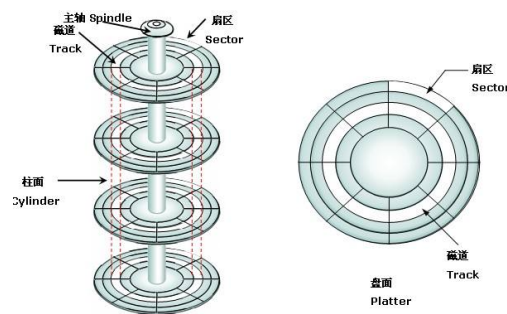
图 23: 机械硬盘结构示意图
