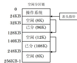
图 10: 空闲分区链
