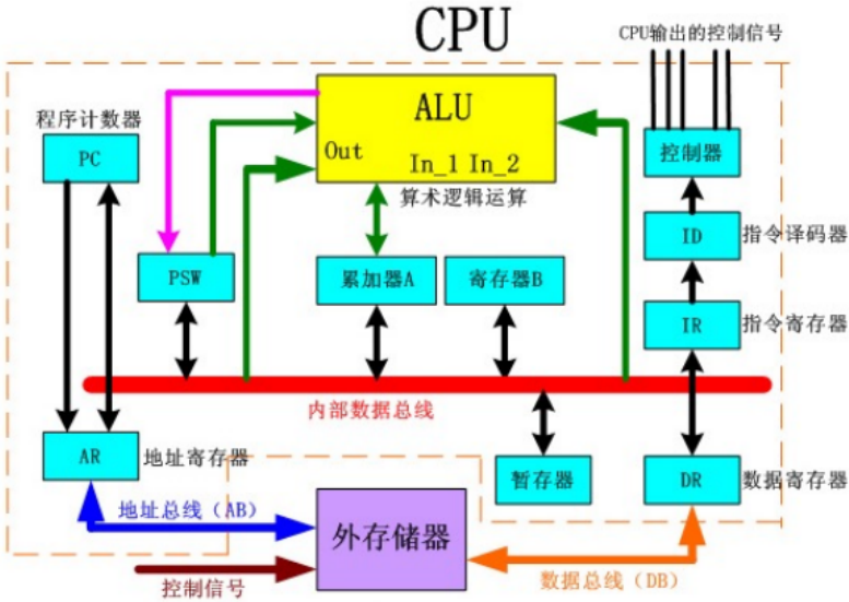
图 1: CPU 重要寄存器示意图
