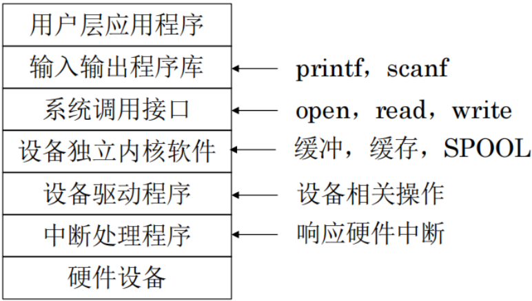
图 26: I/O 系统层次架构示意图
