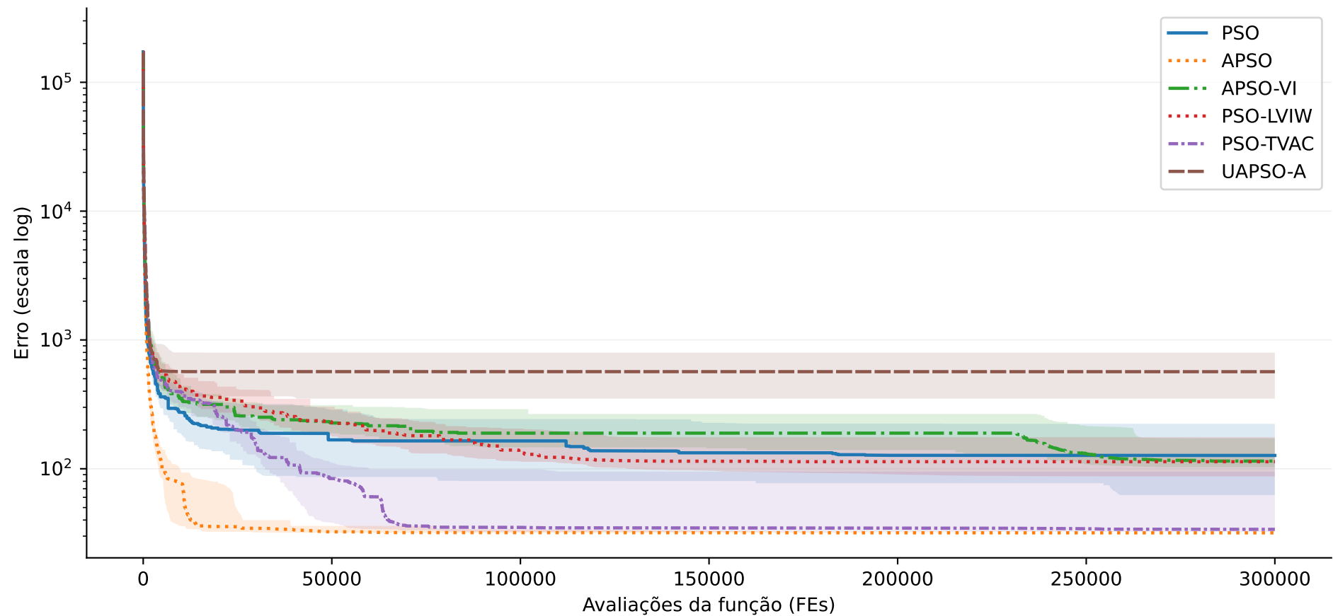
F3 — Zakharov, Dim: 30
