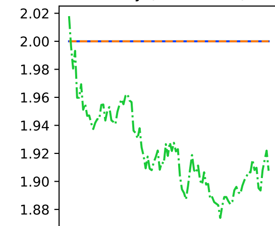
Ackley (dim = 500)
