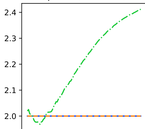
Sphere (dim = 50)
