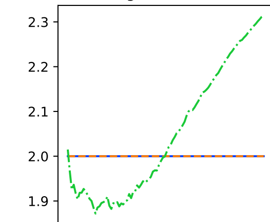
Rastrigin (dim = 500)
