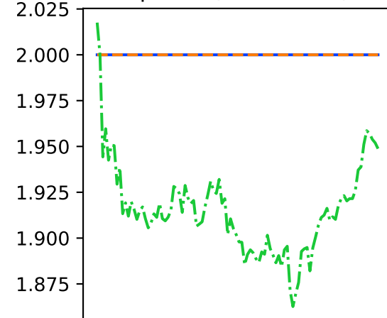
Sphere (dim = 500)
