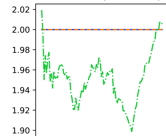
Rosenbrock (dim = 500)
