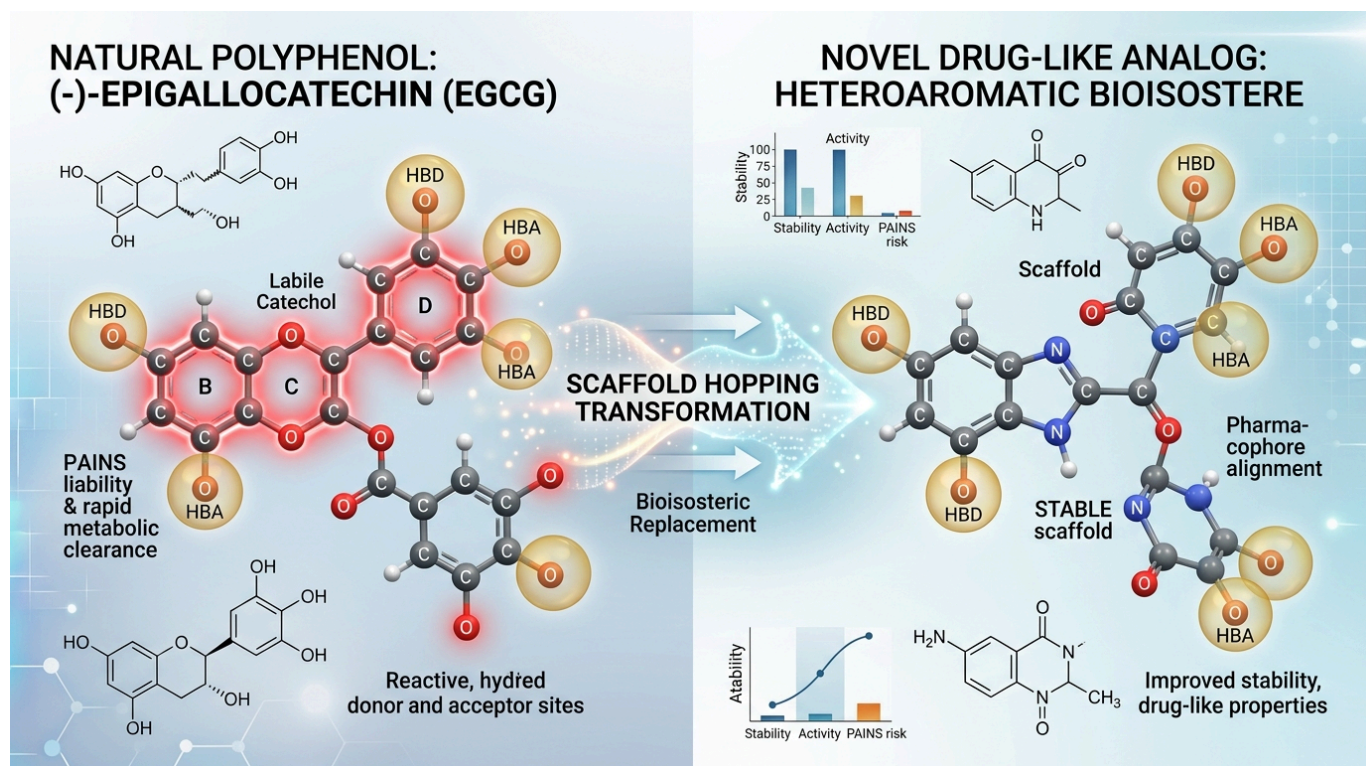
Obrázek 2: 3D Scaffold Hopping z (-)-Epigallocatechinu (EGC): Transformace labilního přírodního polyfenolu na stabilní heteroaromatický bioisoster se zachováním farmakoformní triády. Vlevo: Přírodní polyfenol EGC s vyznačením reaktivního katecholového a pyrogallolového kruhu podléhajících autoxidaci a rychlé jaterní clearance. Vpravo: De novo navržený stabilní bioisoster, v němž byly labilní fenolické kruhy nahrazeny pyridonovým a benzimidazolovým jádrem při striktním zachování prostorových vektorů donorů (HBD) a akceptorů (HBA) vodíkových vazeb.
