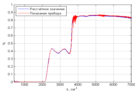
Рисунок 9 - Коэффициент пропускания стекла
