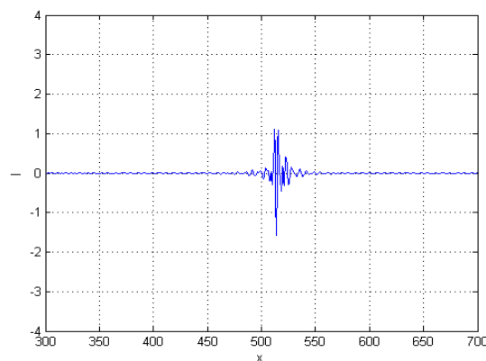
Рисунок 4 - Экспериментально полученная интерферограмма для стекла с напылением \text{CuO}
