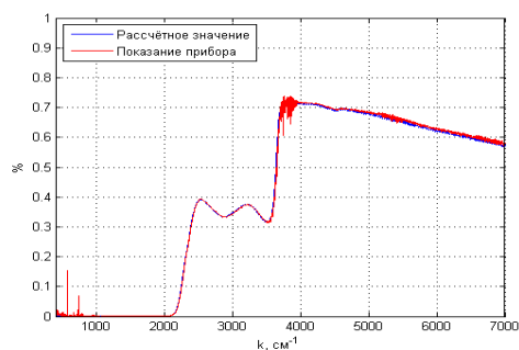
Рисунок 10 - Коэффициент пропускания стекла с напылением CuO
