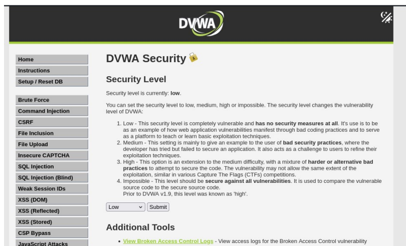
Рисунок 4.2: Запуск DVWA
