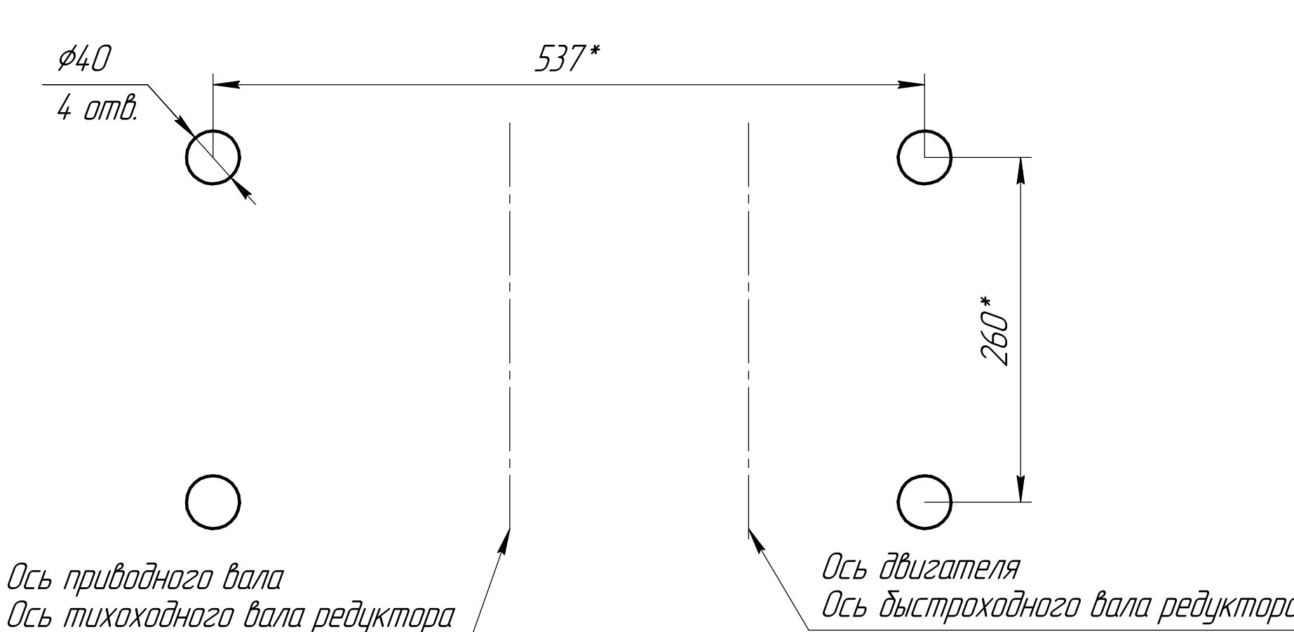
План размещения отверстий под фундаментальные болты
