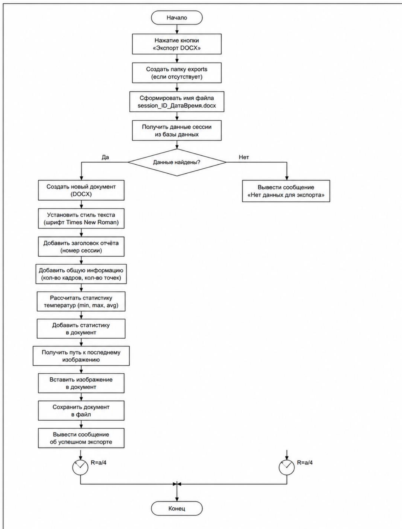
Рисунок 3.3 – Блок-схема алгоритма экспорта в файл в формате DOCX
