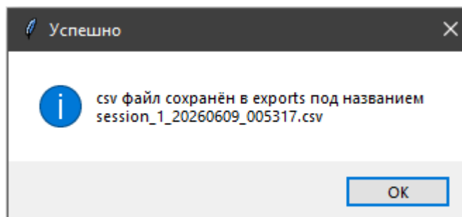
Рисунок 4.4 – Успешный экспорт
