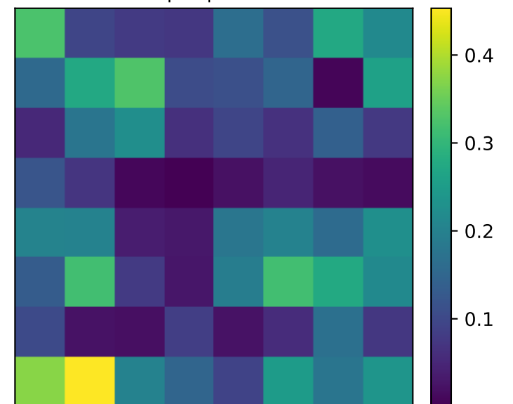
|\text{Err}| t=5
