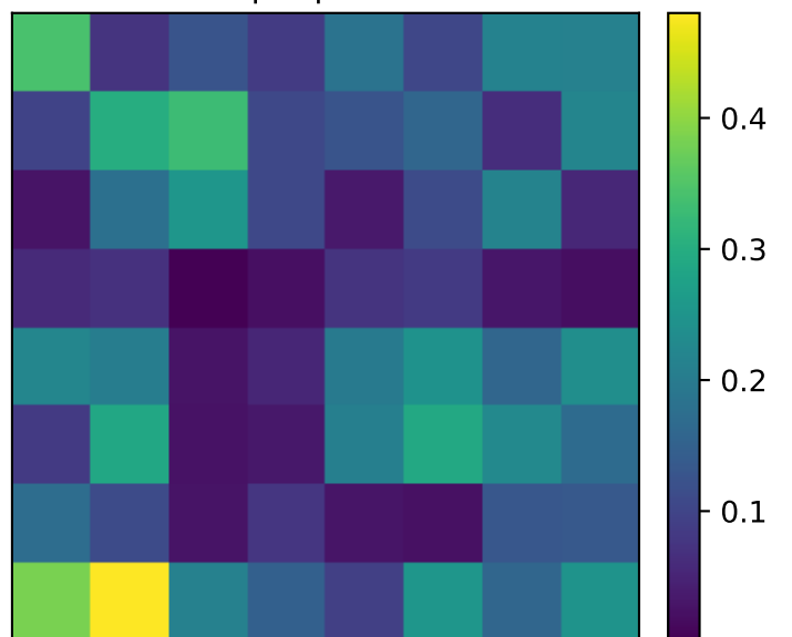
|\text{Err}| t=0
