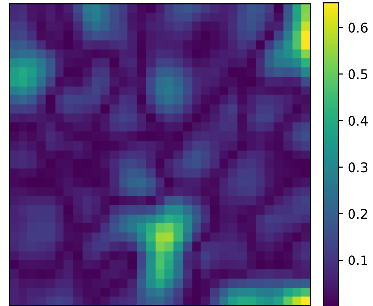
|Pred-GT|/|GT|
