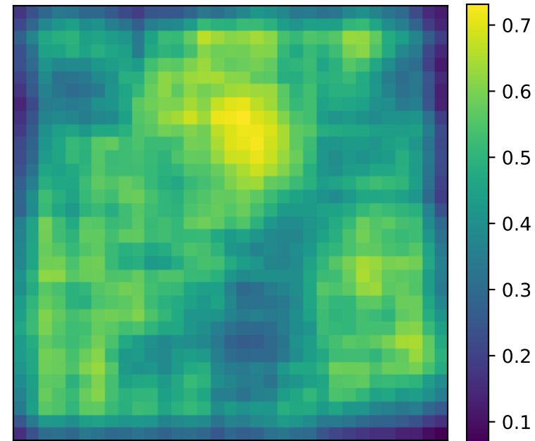
input
