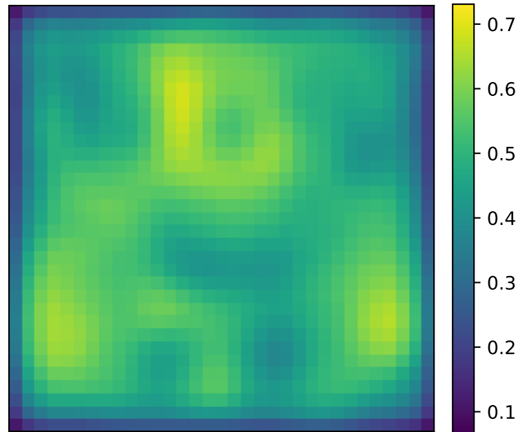
Pred
