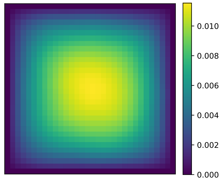
Pred
