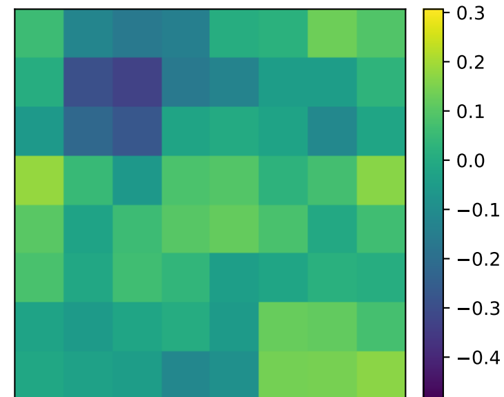
Pred t=5
