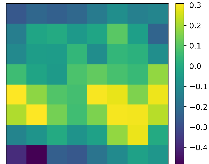
GT t=5
