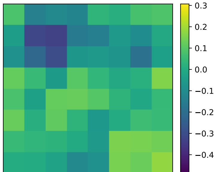
Pred t=0
