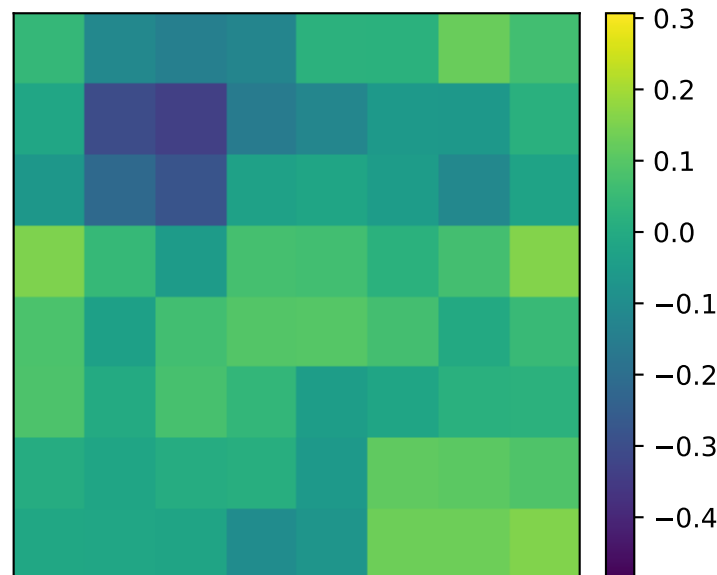
Pred t=3
