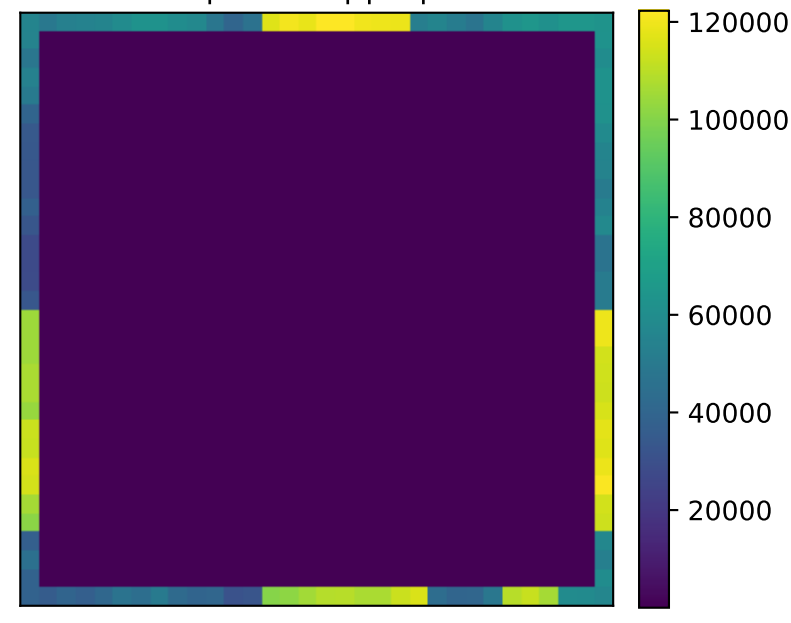
|Pred-GT|/|GT|
