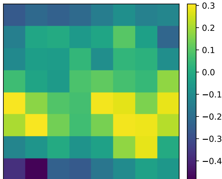
GT t=0
