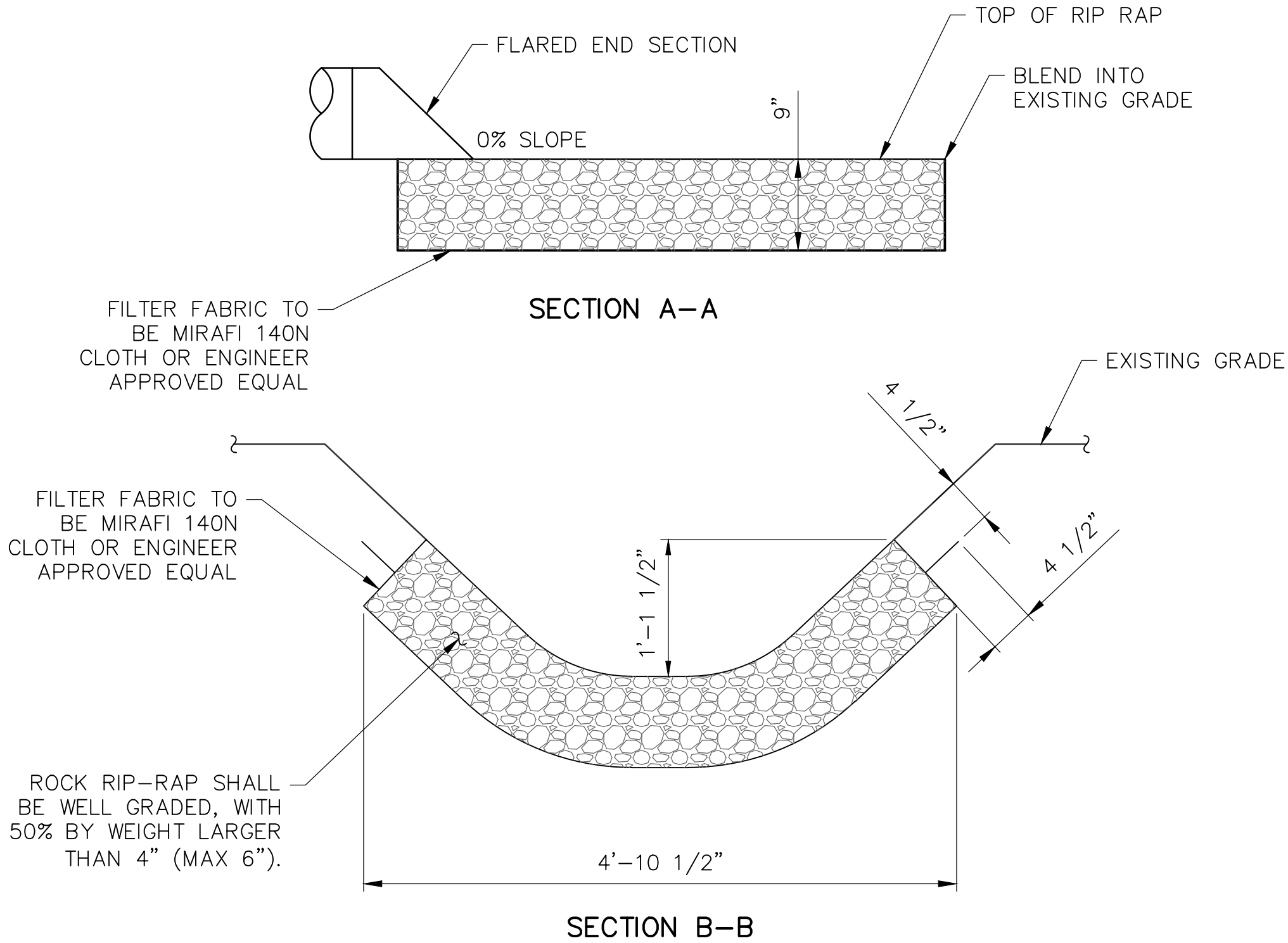
3 OUTLET PROTECTION SCALE: 1/2" = 1'-0" (11x17 SIZE) 1" = 1'-0" (22x34 SIZE)
