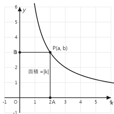
圖：P(a, b) 在圖像上
