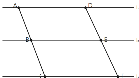
圖： l_1 \parallel l_2 \parallel l_3 ， AB:BC = DE:EF
