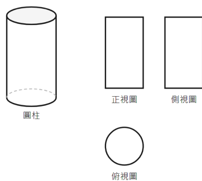
圖：圓柱的三視圖
