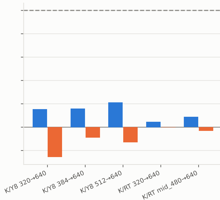
08 detector (KITTI, mono)
