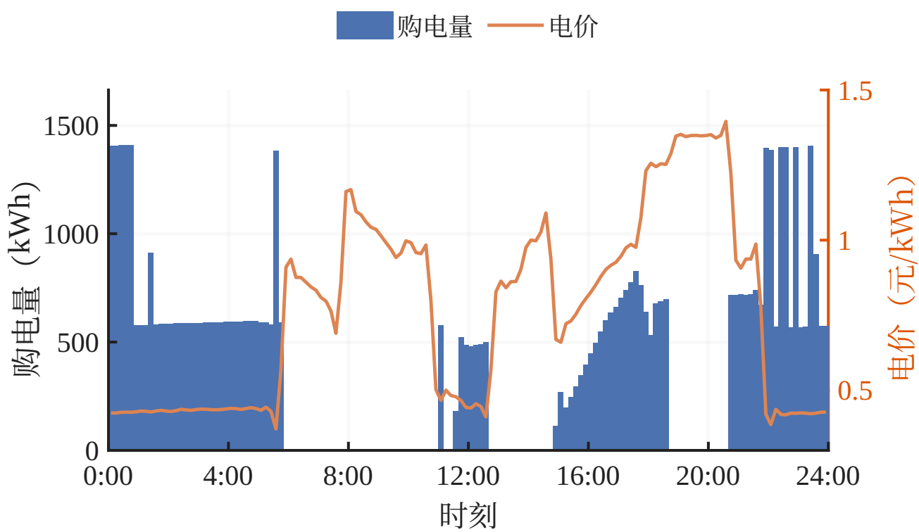
典型日计划购电策略
