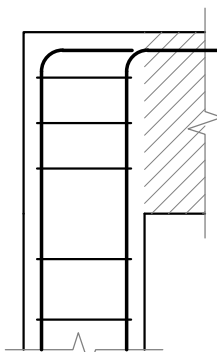
(b) EDGE / CORNER: HOOKS INWARD
