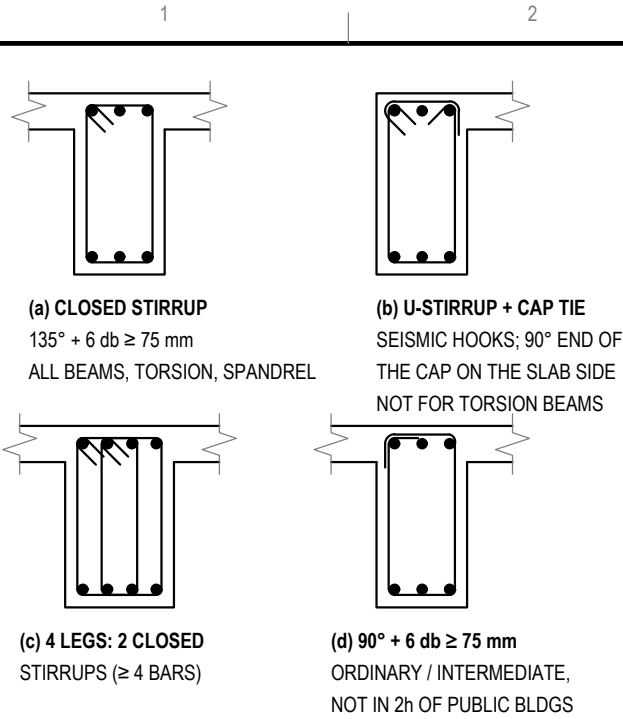
STIRRUP AND HOOP TYPES SCALE N.T.S. 1116
