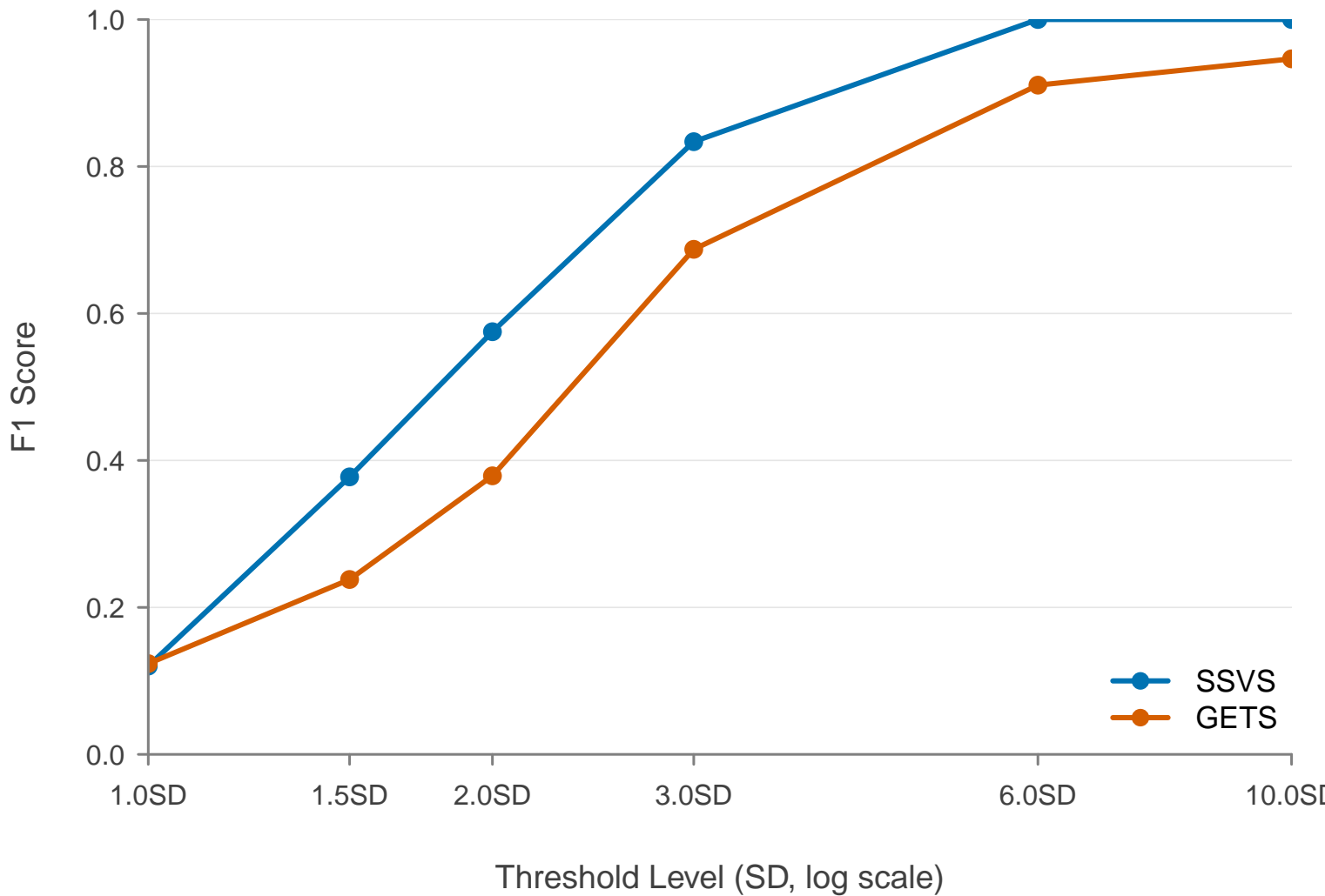
F1 Score Comparison
