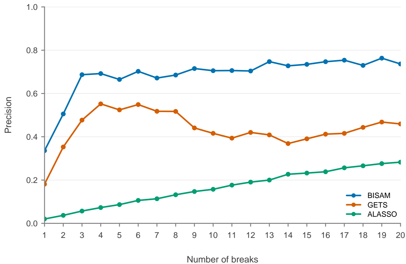
Precision
