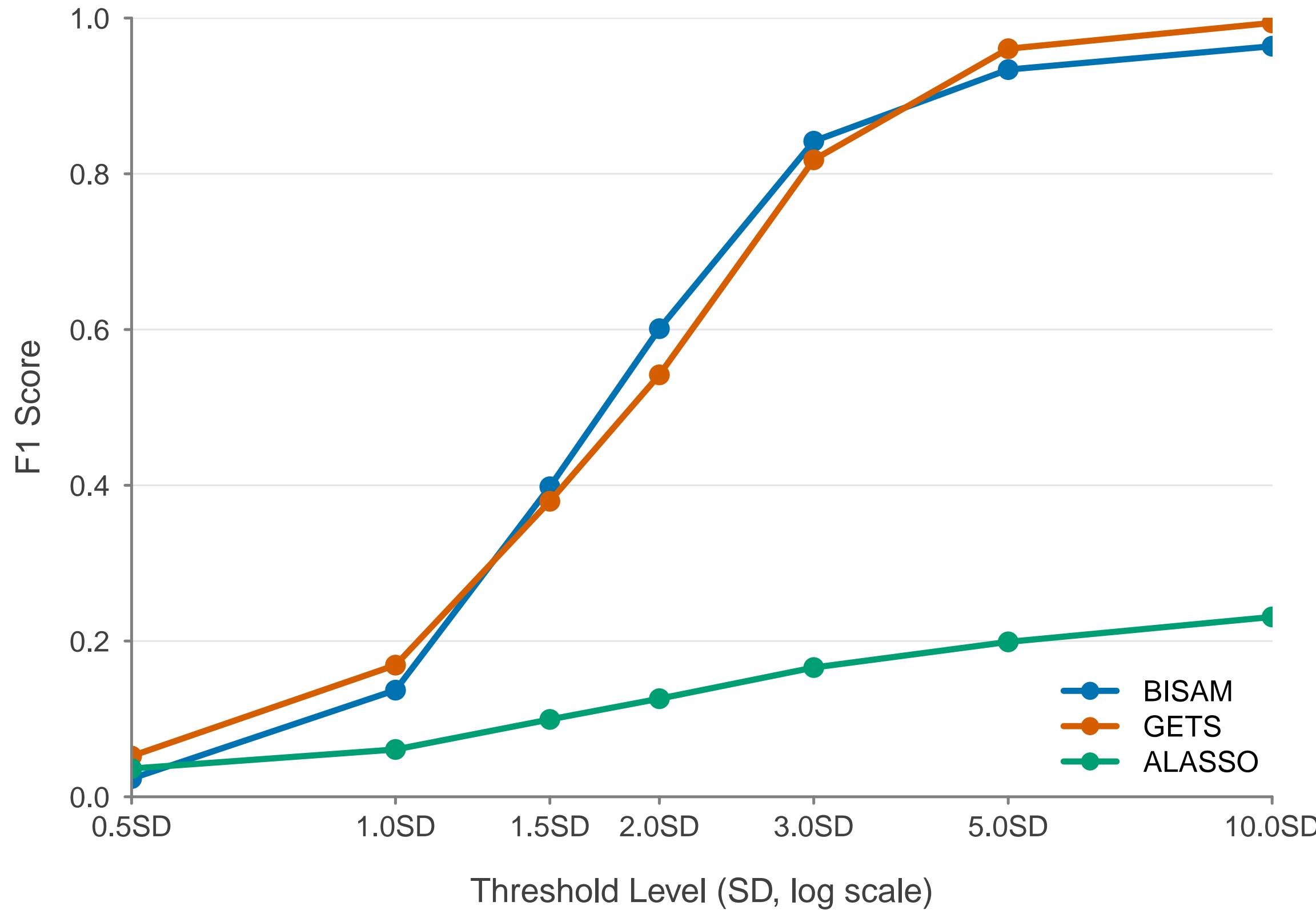
F1 Score
