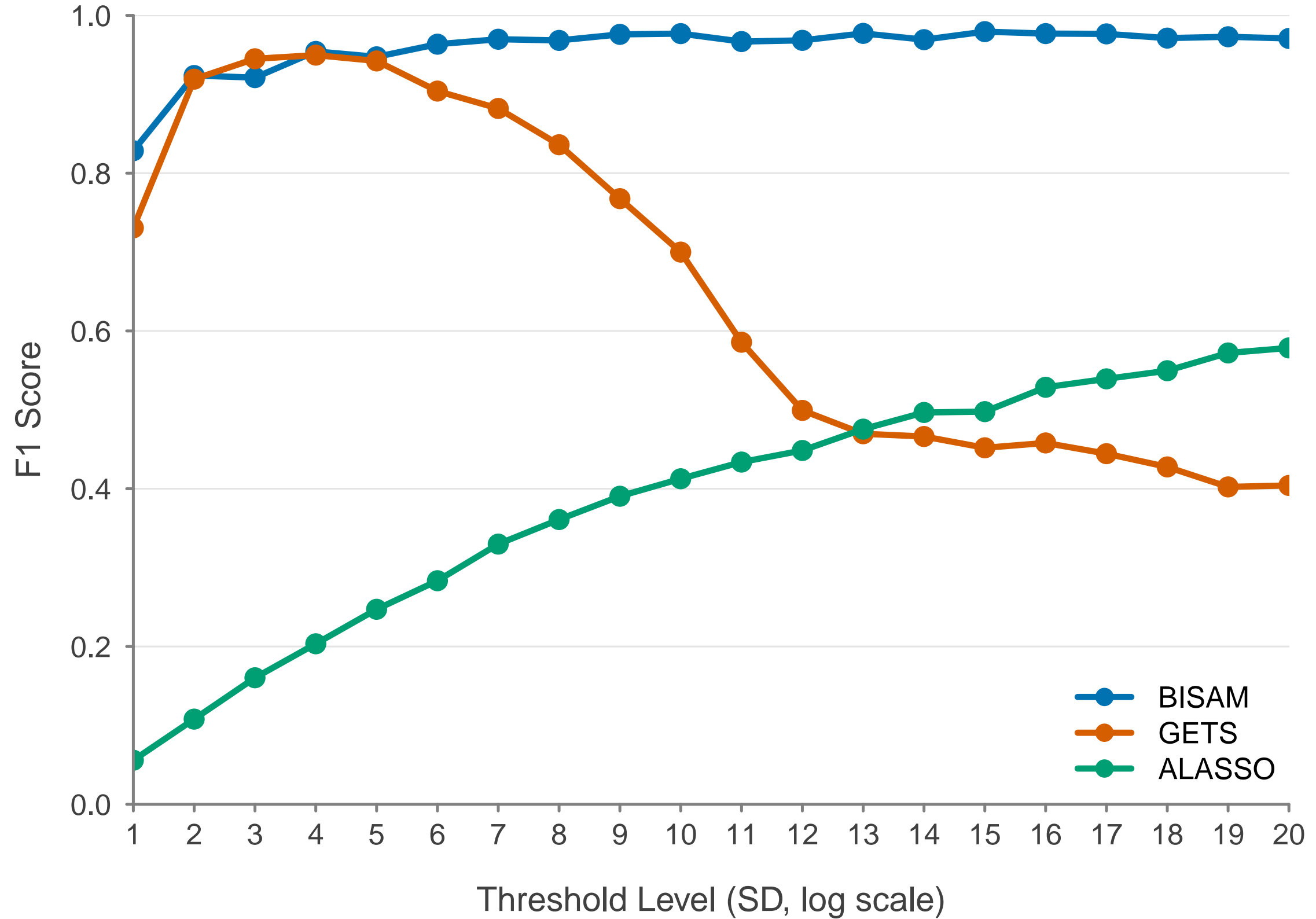
F1 Score
