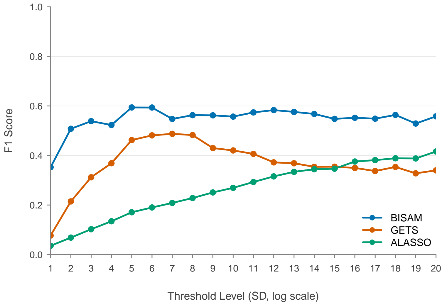
F1 Score
