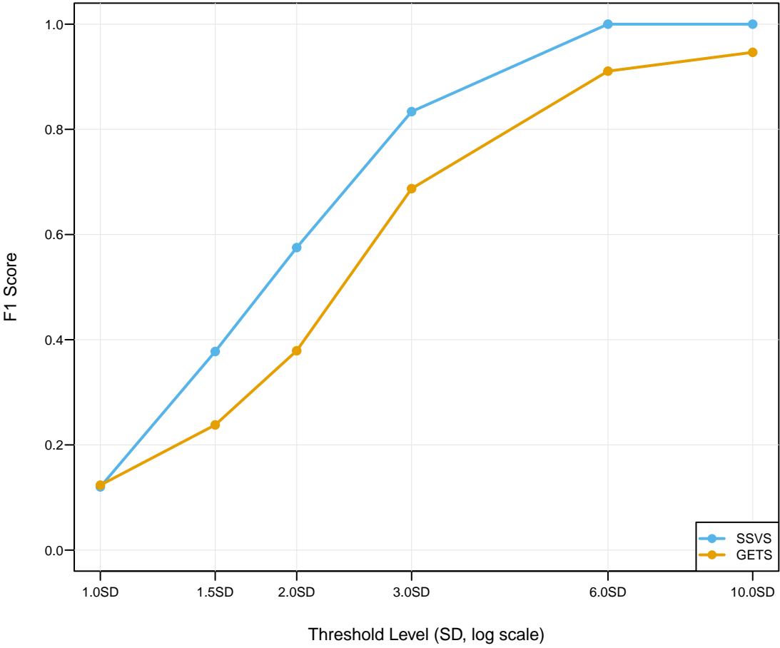
F1 Score Comparison
