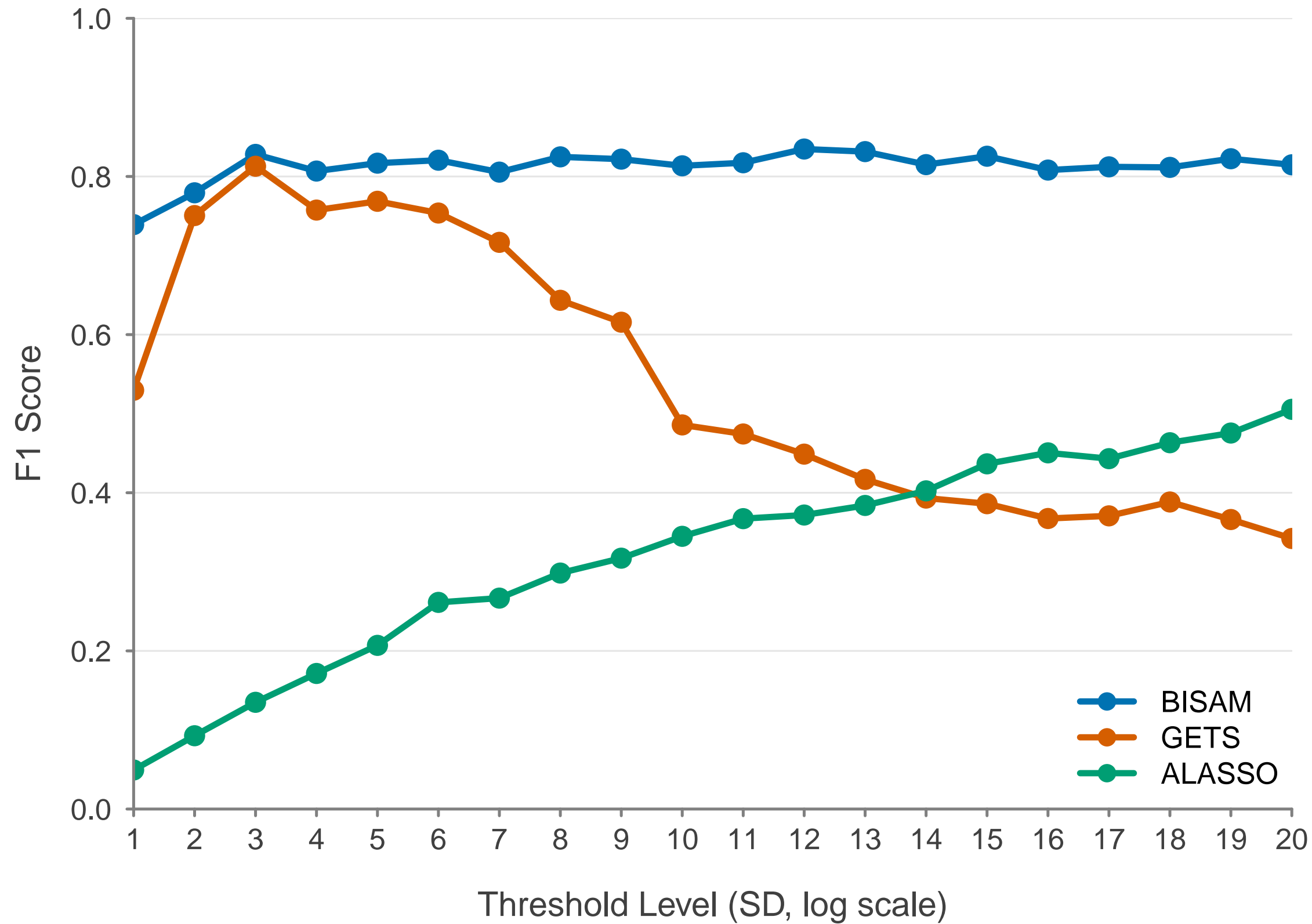
F1 Score
