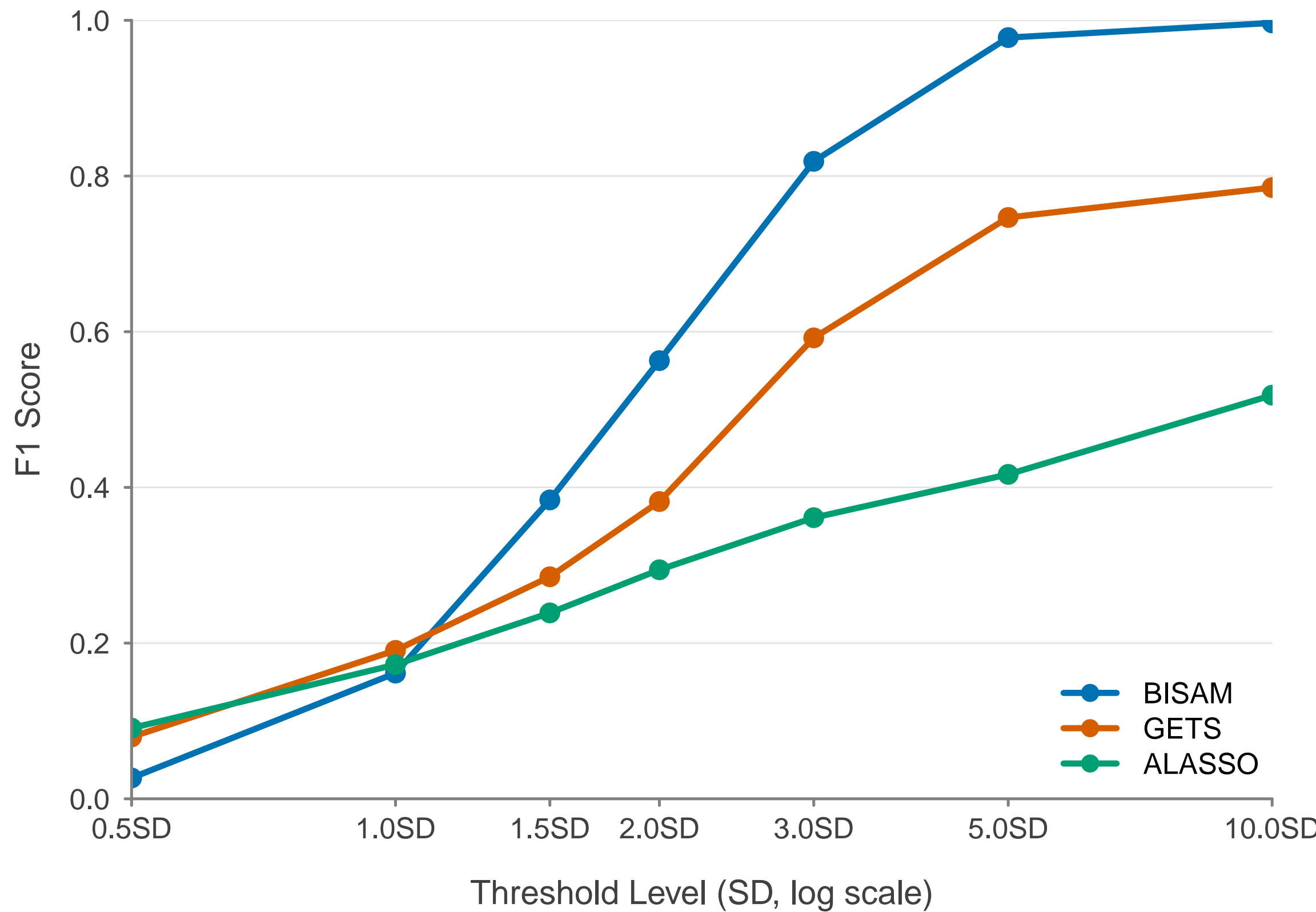
F1 Score
