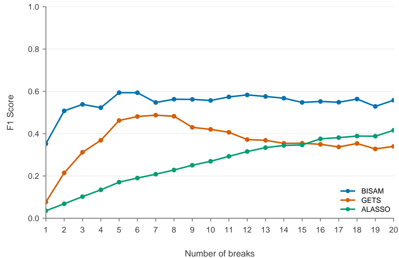
F1 Score
