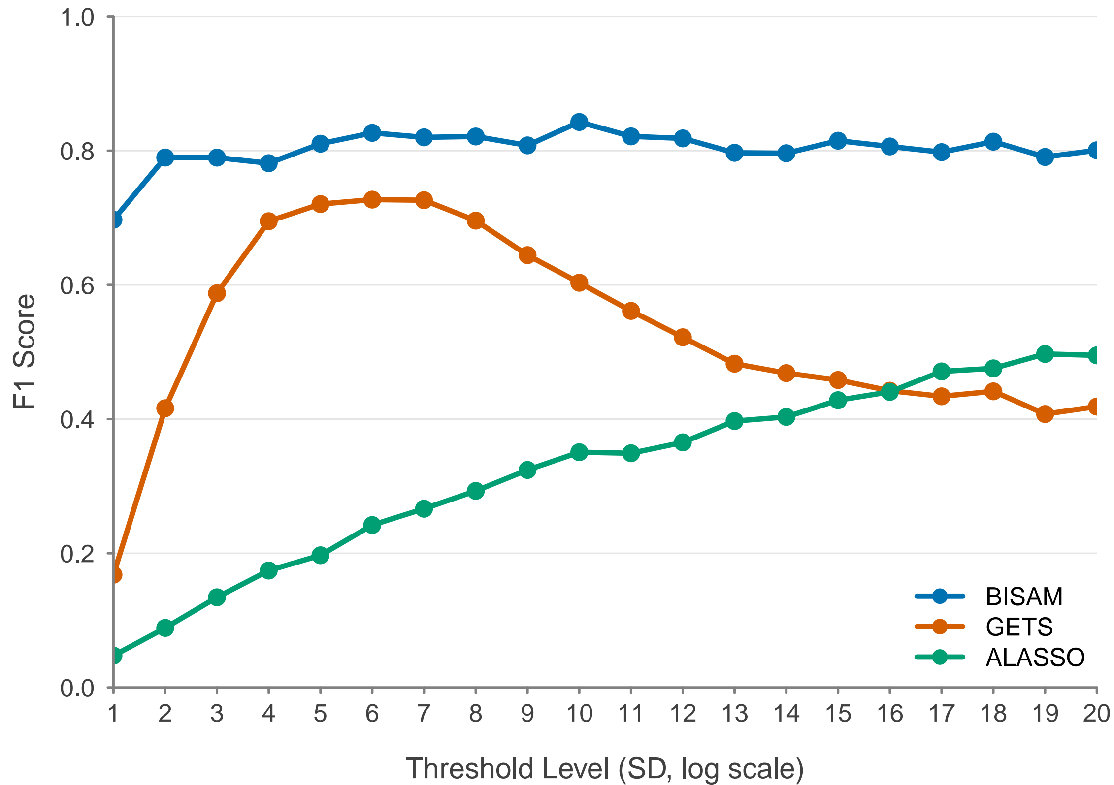
F1 Score
