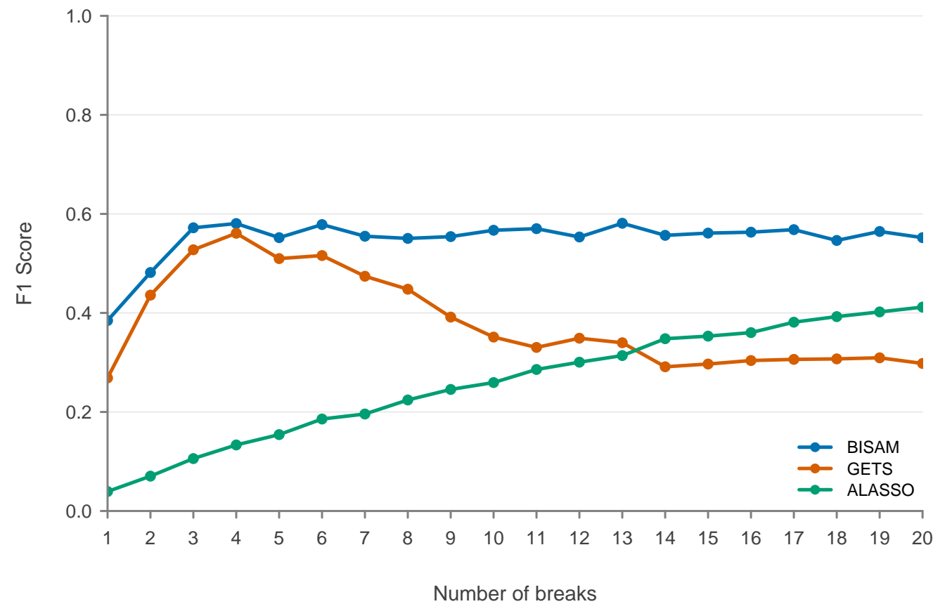
F1 Score
