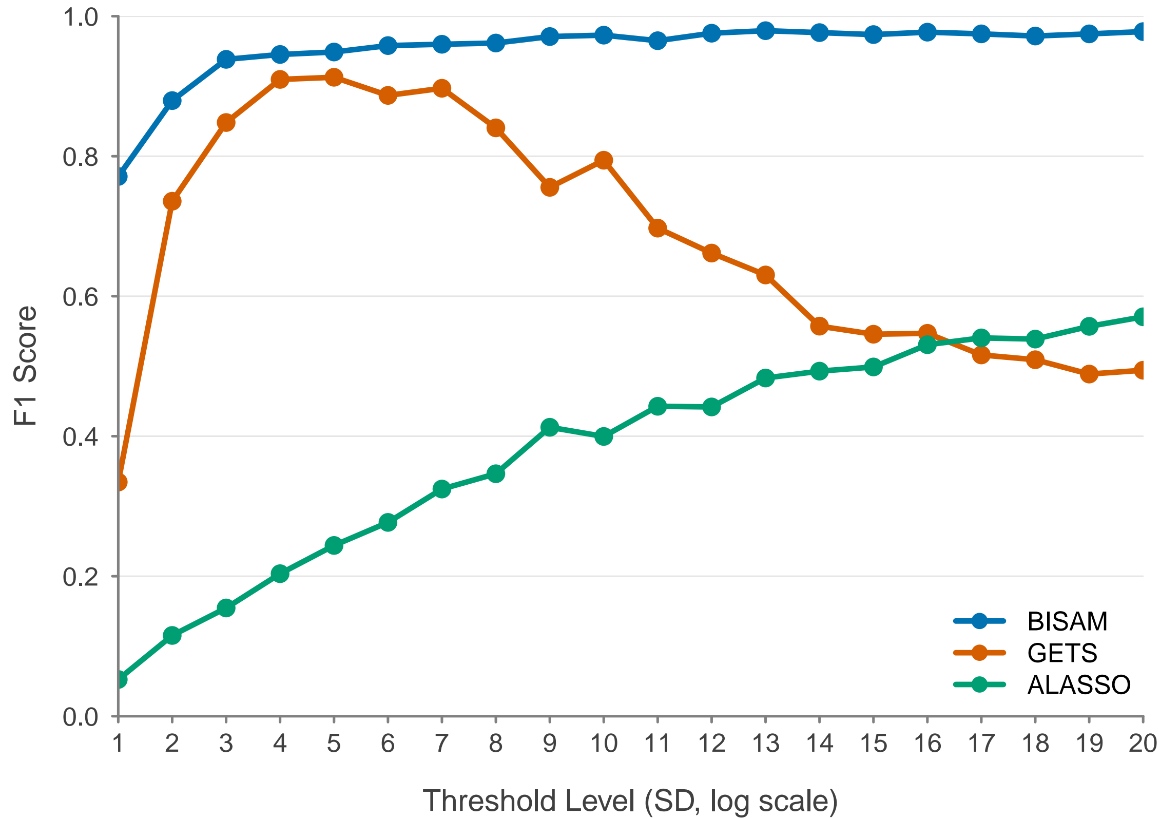
F1 Score
