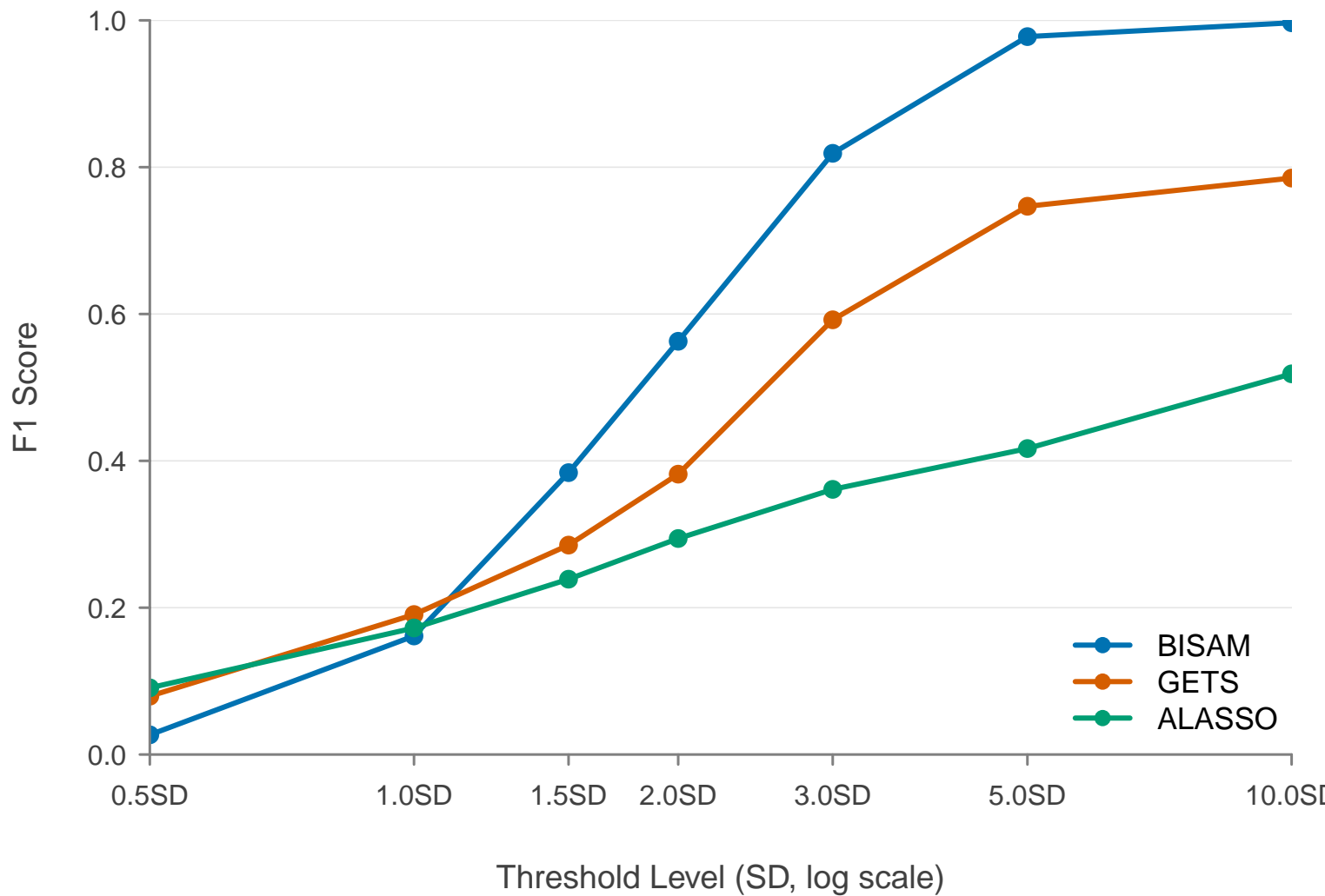
F1 Score
