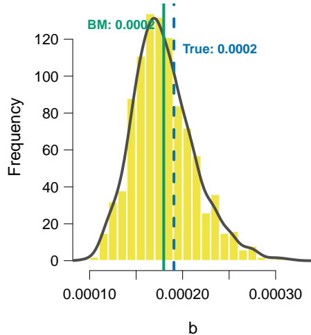
(c) Scale Parameter b
