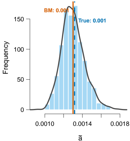
(b) Location Parameter \tilde{a}
