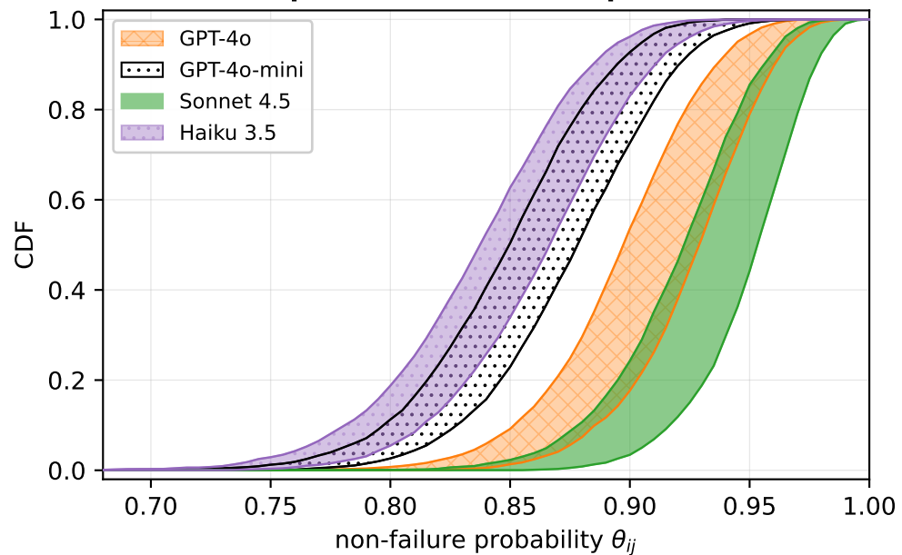
Subdomain posterior CDF envelopes: D2 / RACE-H
