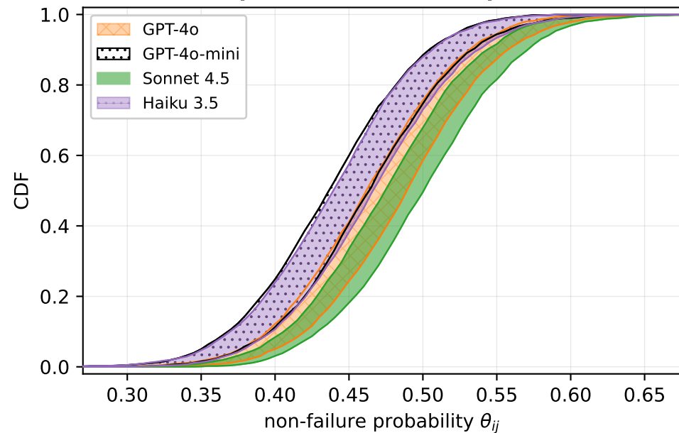
Subdomain posterior CDF envelopes: D1 / MBPP
