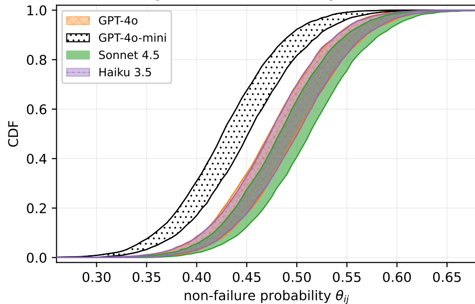
Subdomain posterior CDF envelopes: D1 / DS-1000
