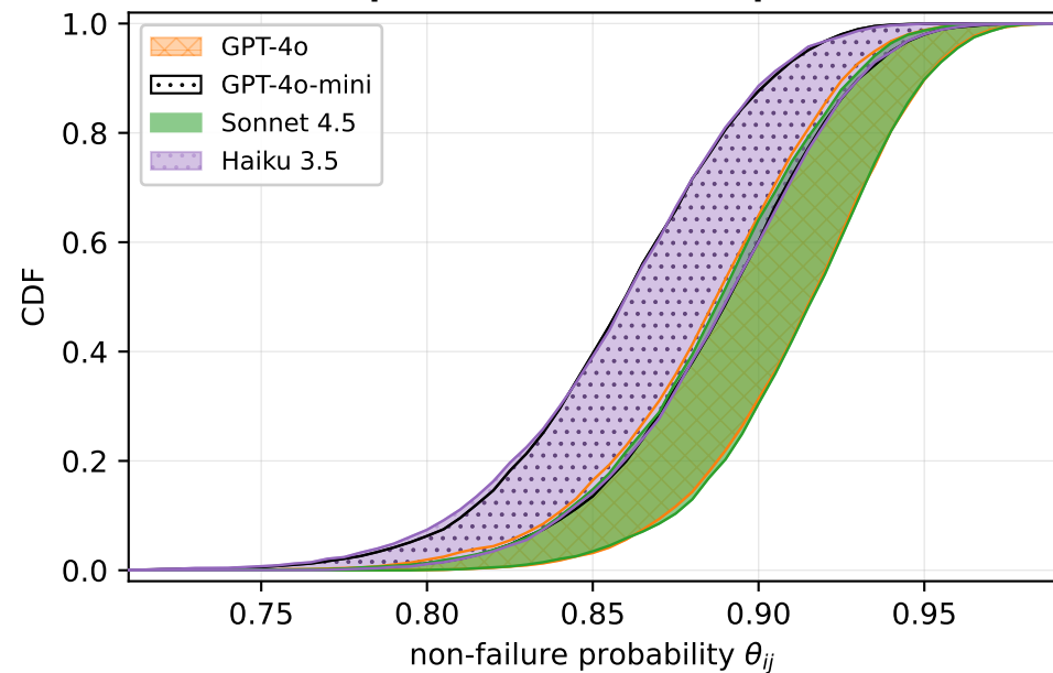
Subdomain posterior CDF envelopes: D2 / BoolQ
