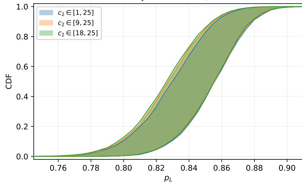
Narrowing the c_2 prior range (LLM-level posterior CDF, GPT-4o)
