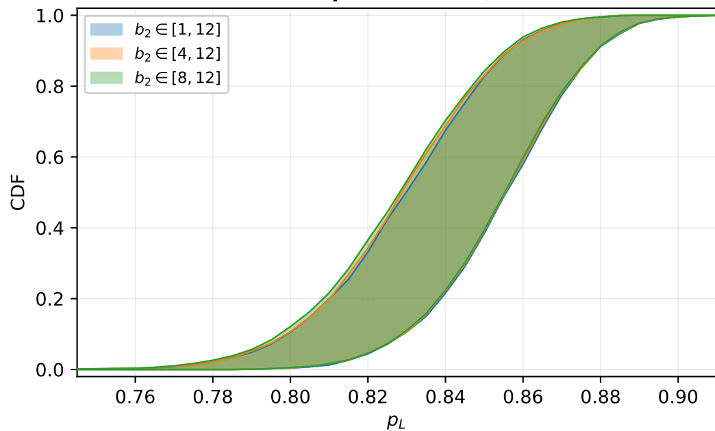
Narrowing the b_2 prior range (LLM-level posterior CDF, GPT-4o)
