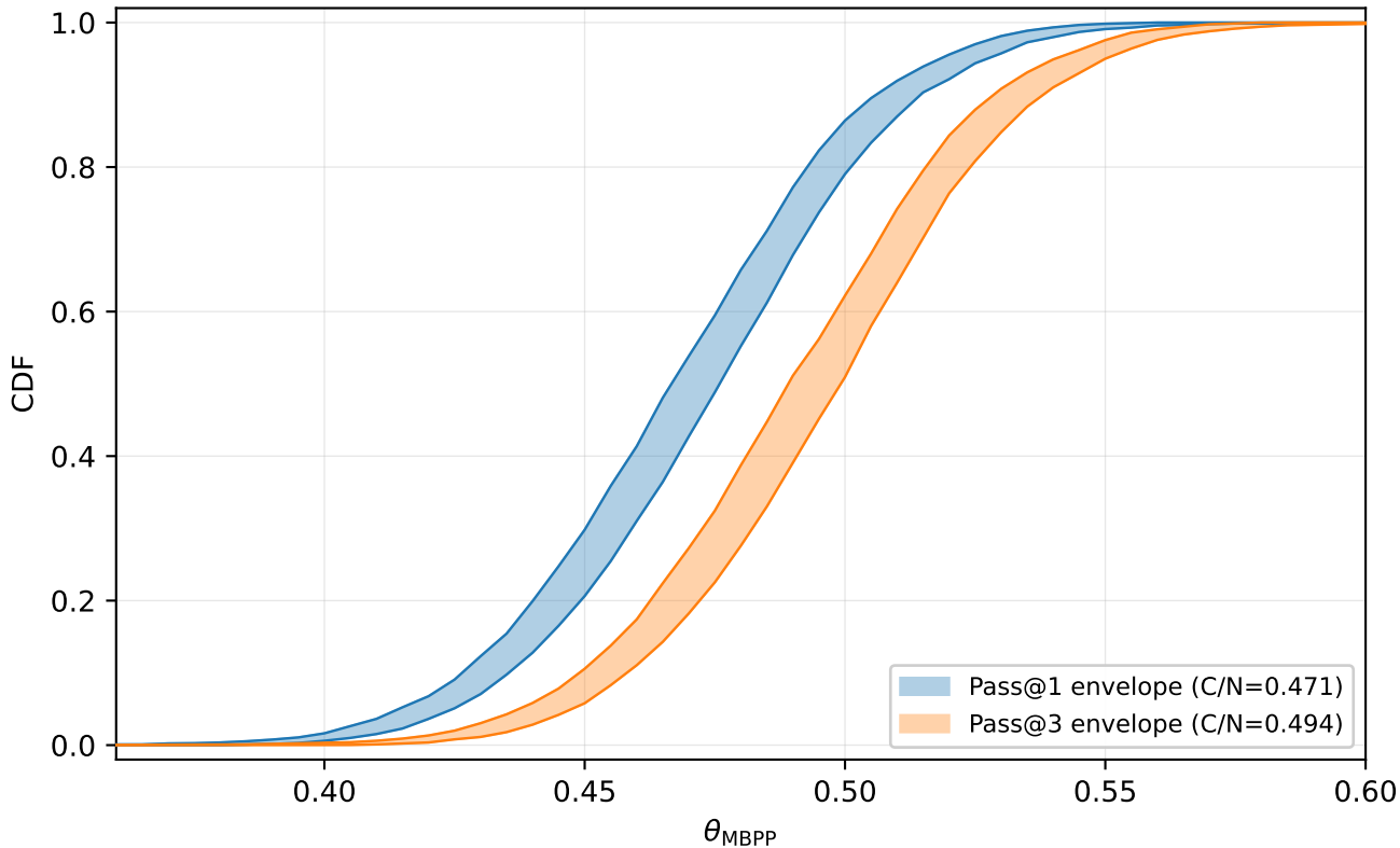
Subdomain posterior CDF envelopes: MBPP - Pass@1 vs Pass@3
