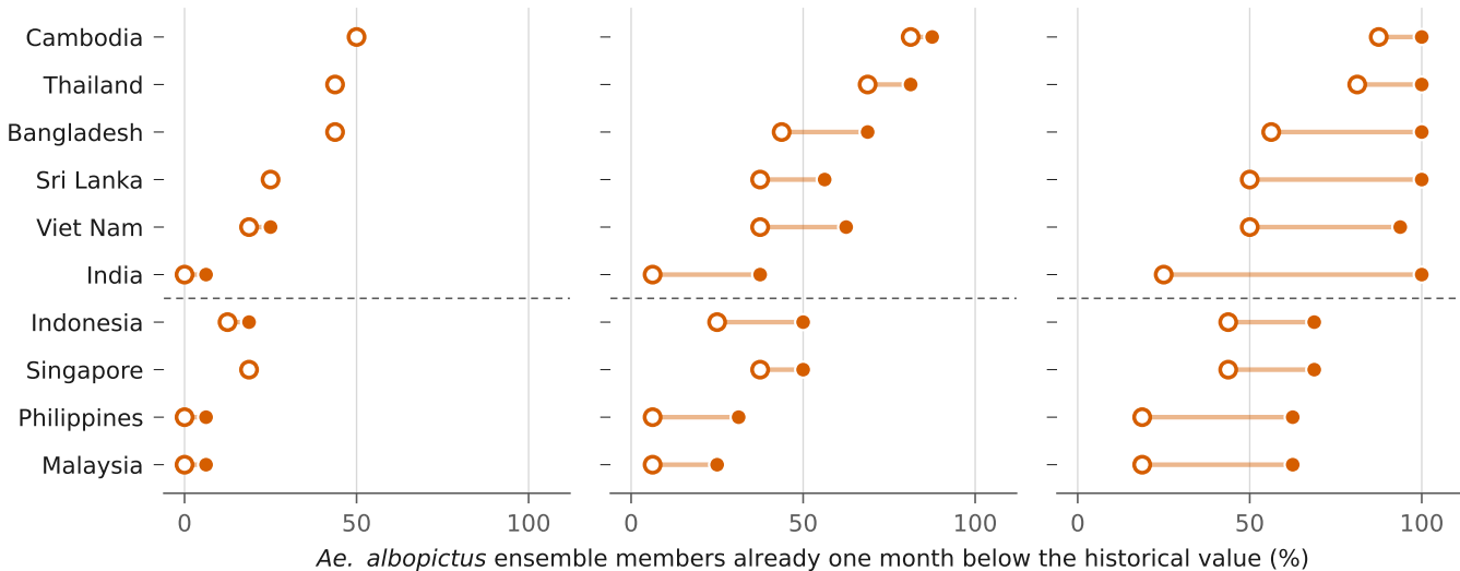
SSP1-2.6
