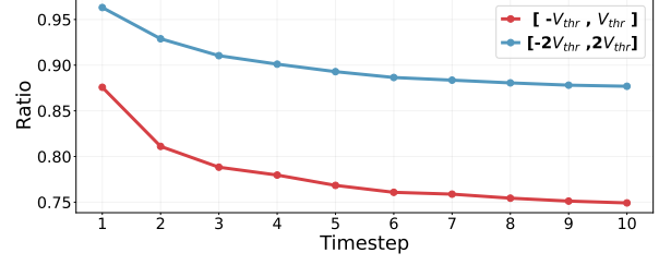
(b) DVS-CIFAR10
