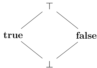
그림 12: Boolean 요약도메인
