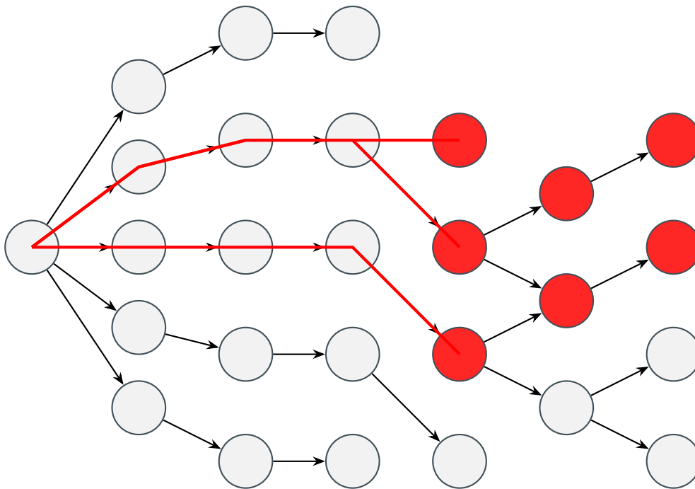
그림 1: Propagation of abstract states through the CFG.
