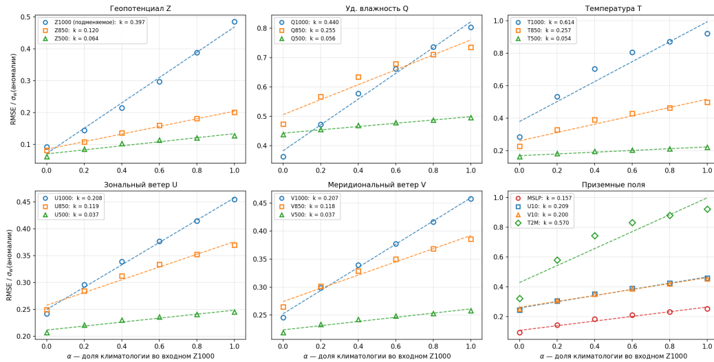
Рис. A8: Pangu-Weather на +24 ч, те же даты и дозы, что на рис. A7. Наклон T1000 растет до 0.614, T2M — до 0.570. У Auroга отклик ослабевает при том же изменении срока, поэтому модели различаются по масштабу и зависимости от заблаговременности.
