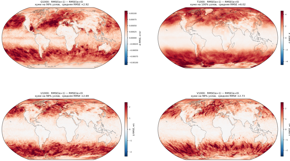
Рис. A10: Ауорога после полной замены Z1000 ( \alpha = 1 , +6 ч; 48 дат 2024 года). Каждая карта показывает временную RMSE измененного прогноза минус временную RMSE базового прогноза в том же узле. Красный цвет означает добавленную ошибку, а не знаковое смещение прогноза. Для T1000 отношение средних по узлам RMSE равно 6.02\times , рост охватывает почти всю сетку.
