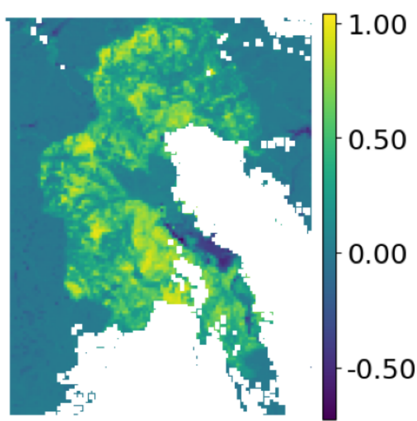
NBR
