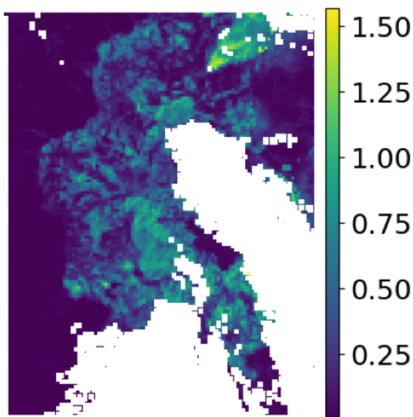
Cosine baseline
