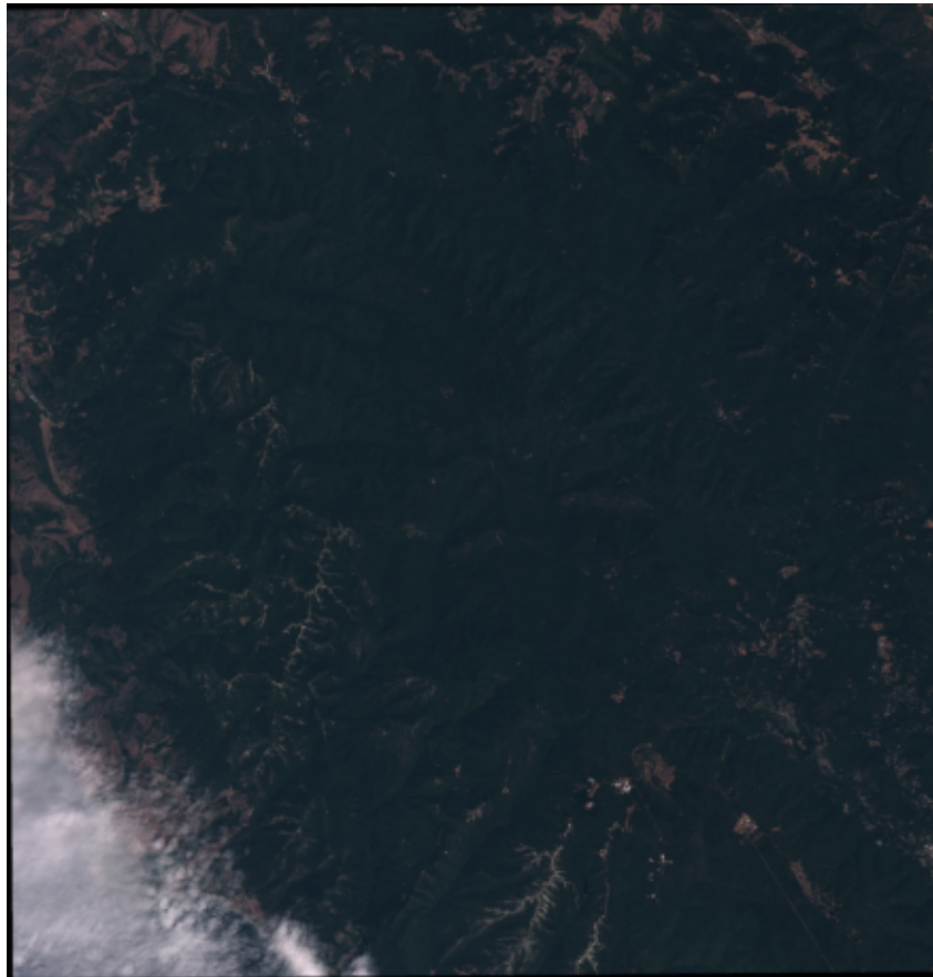
Cosine baseline
