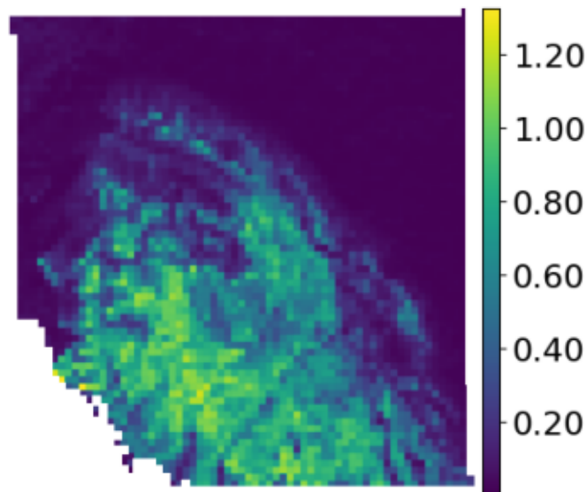
Cosine baseline
