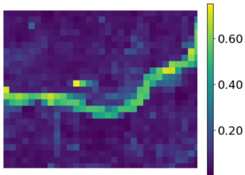
Cosine baseline
