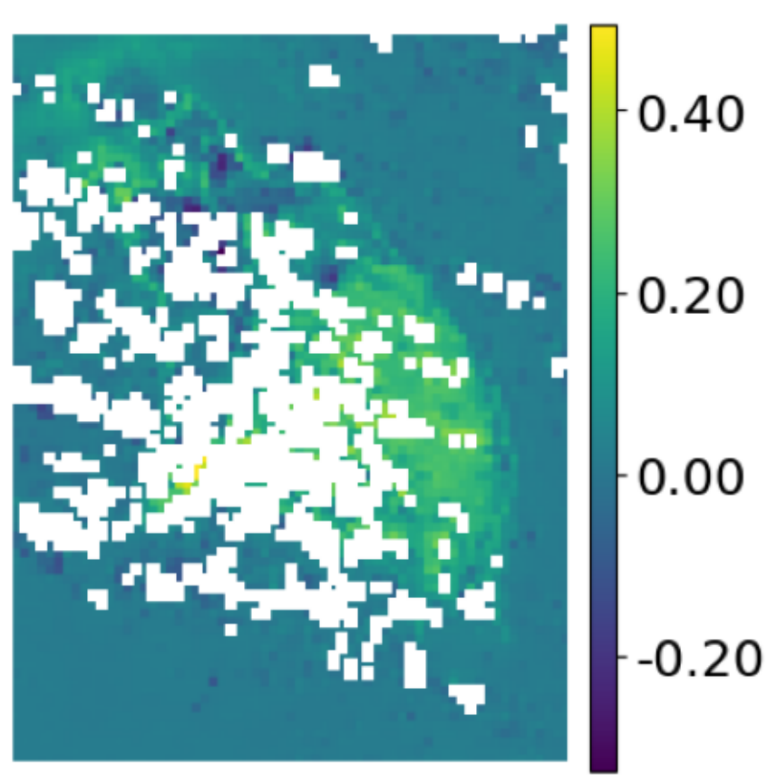
NDVI
