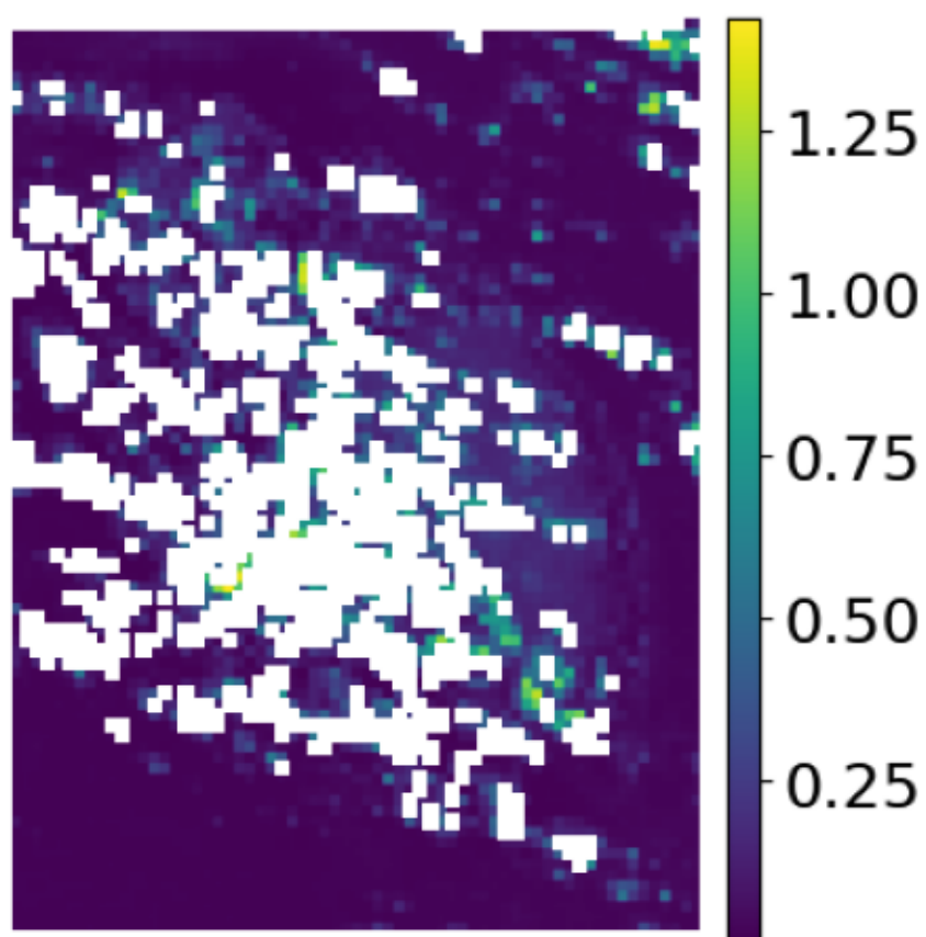
Cosine baseline
