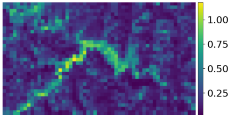
Cosine baseline
