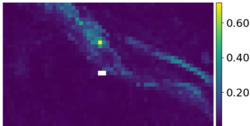
Cosine baseline
