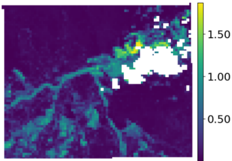
Cosine baseline
